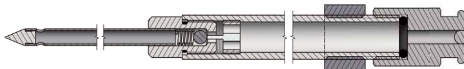
B-STING® Fugeninjektionsnadel, Injektionsrohr mit Gel-Flachkopfnippel | B-STING® игла за инжектиране на фуги, инжекционна тръба с плосък нипел за гел
